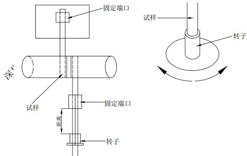
图5 垂直扭转示意图
