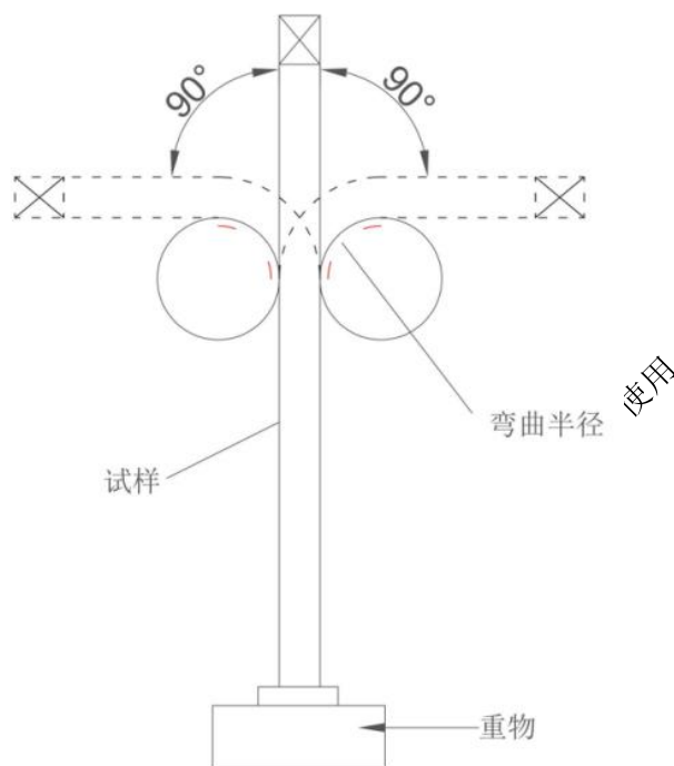
图1 90度摇摆弯曲示意图
