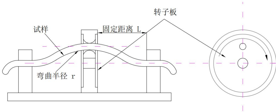
图2 弯折及旋转示意图
