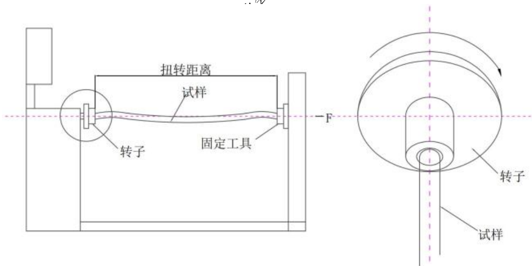
图3 2D 扭转示意图
